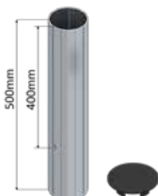
S30357BR-01 - Fourreau alu pour poteau central Ø 90mm.
